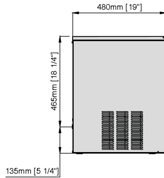
Vue latérale Side view
